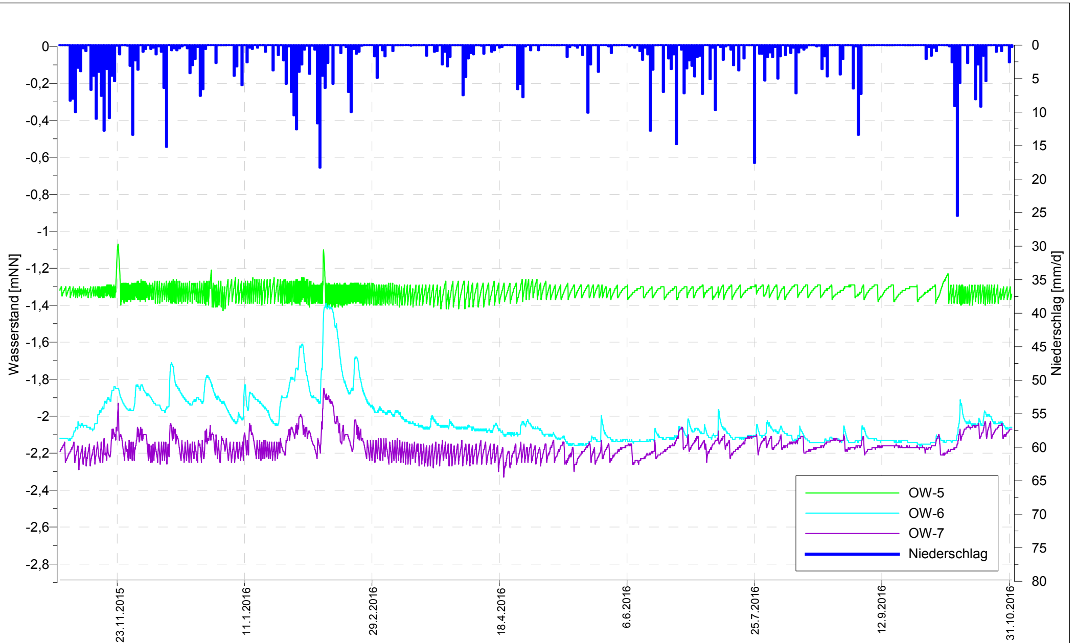
Anl. 4: Wasserstandsganglinien am Oldenburger Graben
