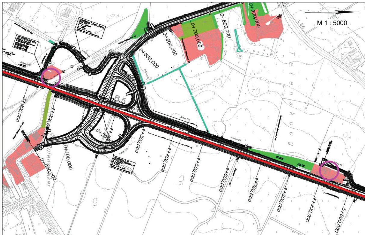
Abbildung 2: Zwangspunkte Trassierung, Teil 2
