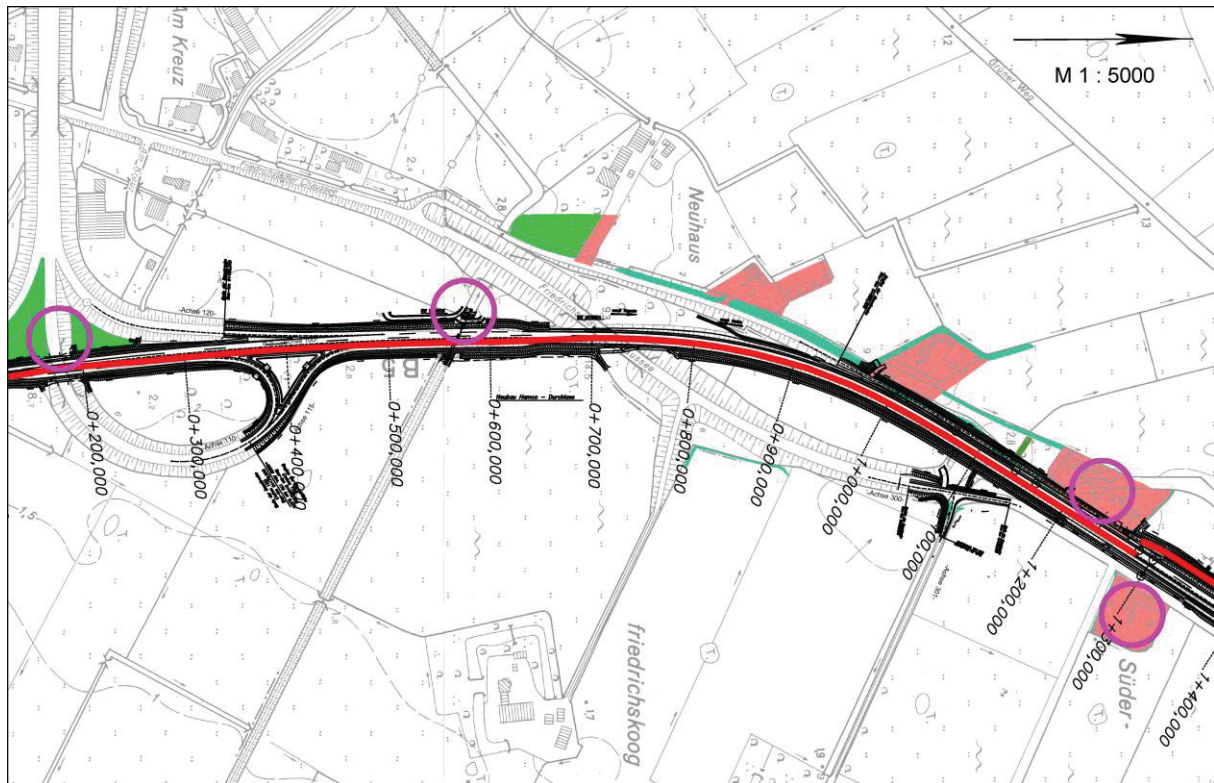
Abbildung 1: Zwangspunkte Trassierung, Teil 1
