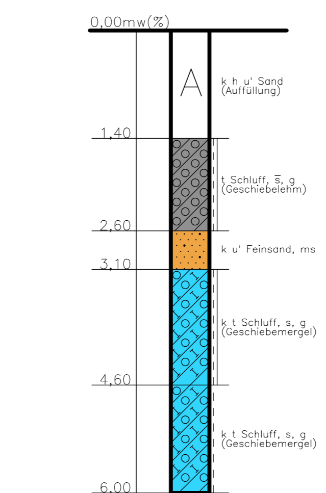
SB 15/159 49+200 / 14m rechts
