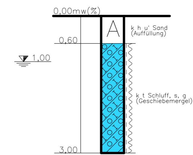
SB 15/158 49+200 / 1,5m rechts
