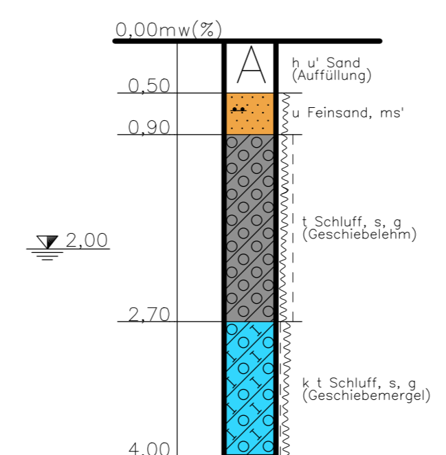
SB 15/155 49+100 / 10m rechts
