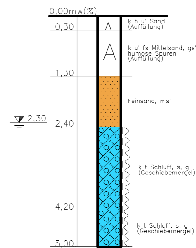
SB 15/150 49+050 / 1,5m rechts
