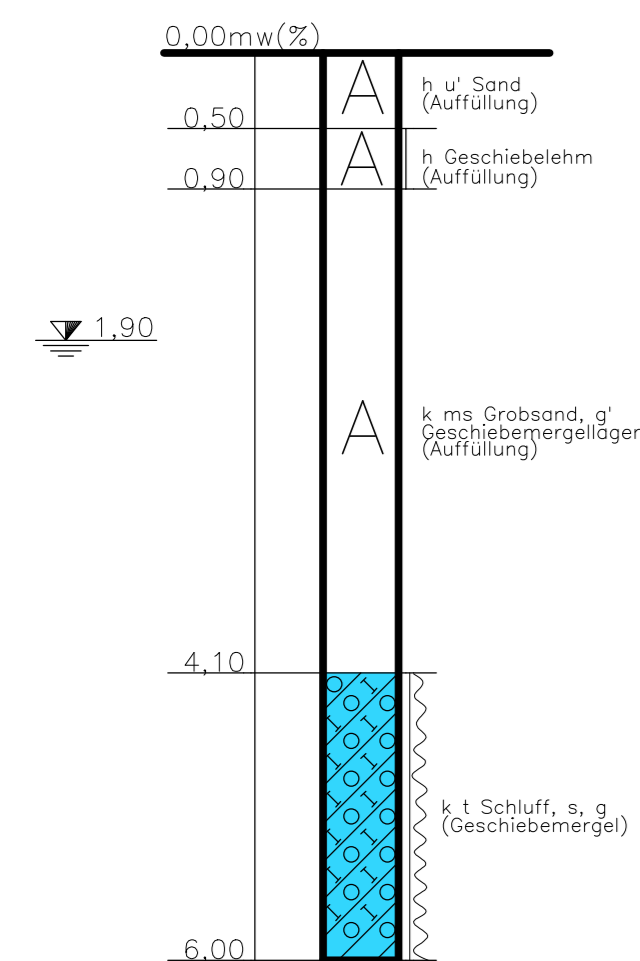
SB 15/145 48+900 / 3m rechts
