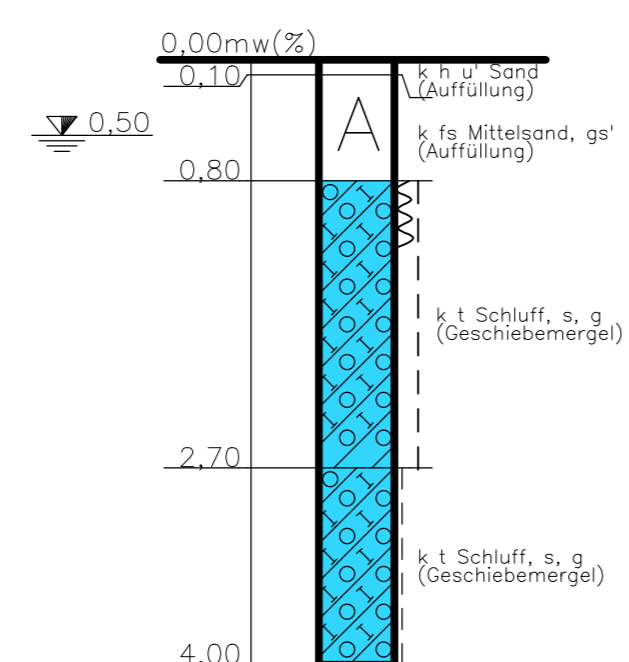
SB 15/148 49+025 / 10m rechts
