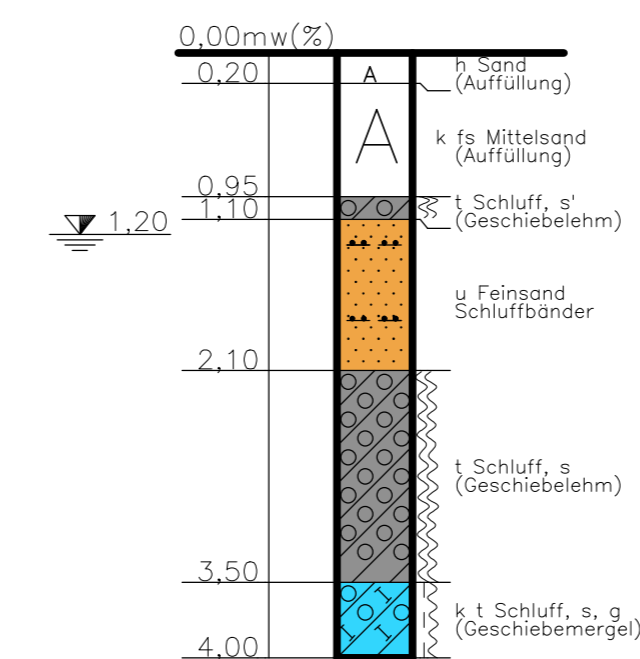
SB 15/156 49+150 / 1,5m rechts
