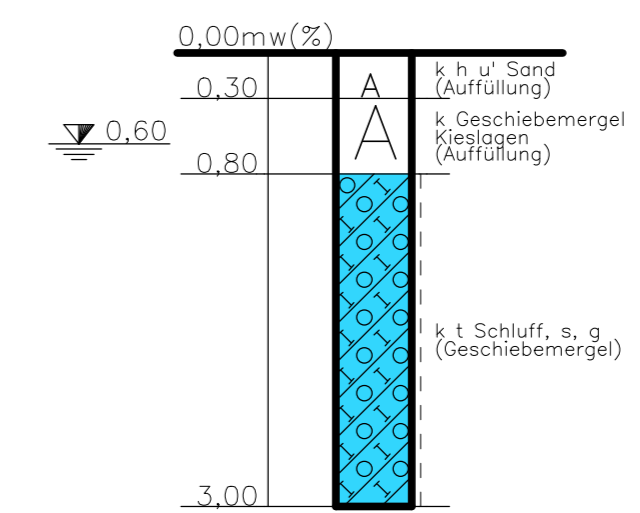
SB 15/160 48+250 / 1,5m rechts
