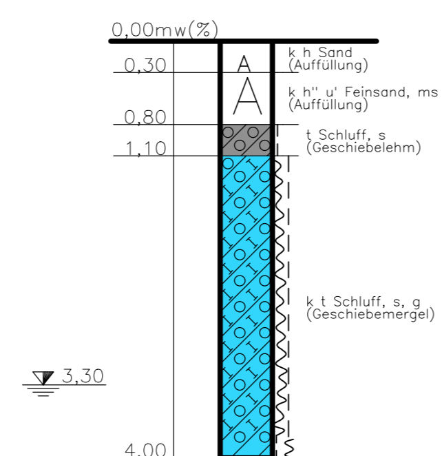
SB 15/151 49+050 / 9m rechts
