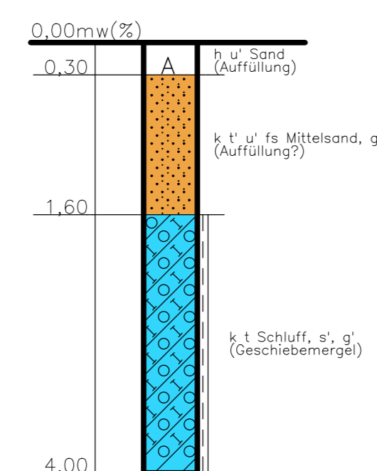
SB 15/147 49+000 / 10m rechts
