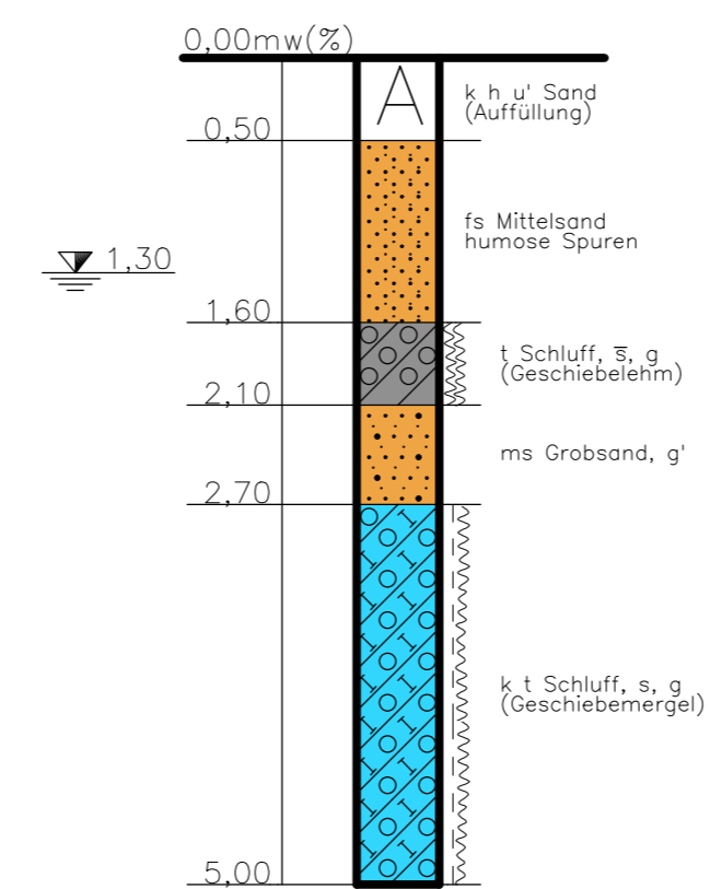
SB 15/154 49+100 / 3m rechts
