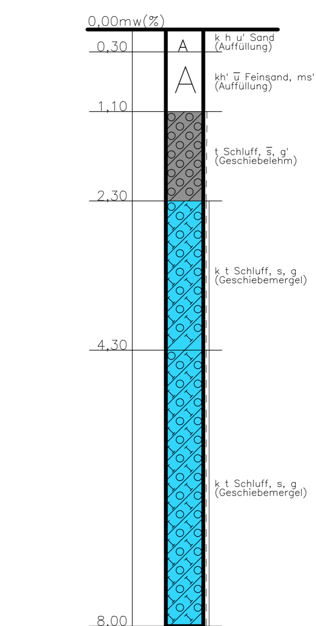
SB 15/161 49+250 / 15m rechts
