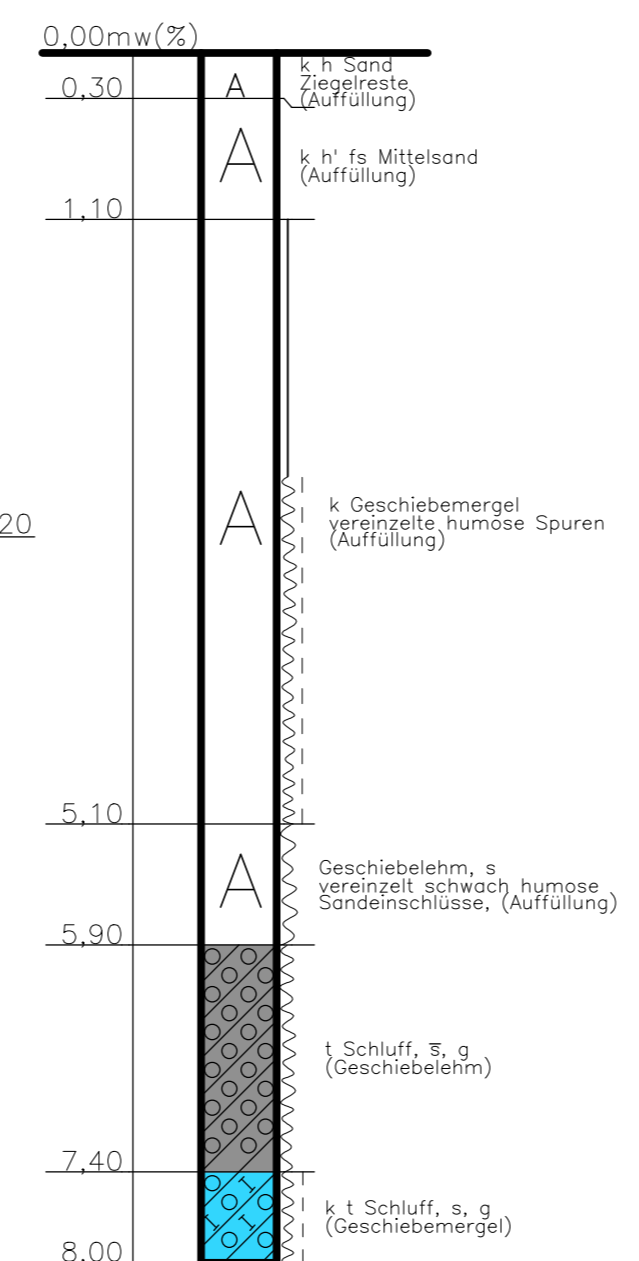
SB 15/153 49+075 / 9m rechts
