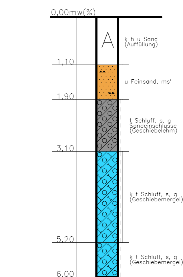
SB 15/157 49+150 / 10m rechts
