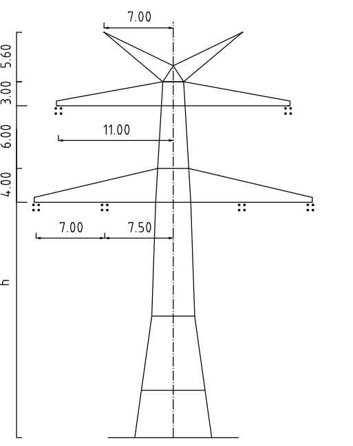
Mast Nr. 004
