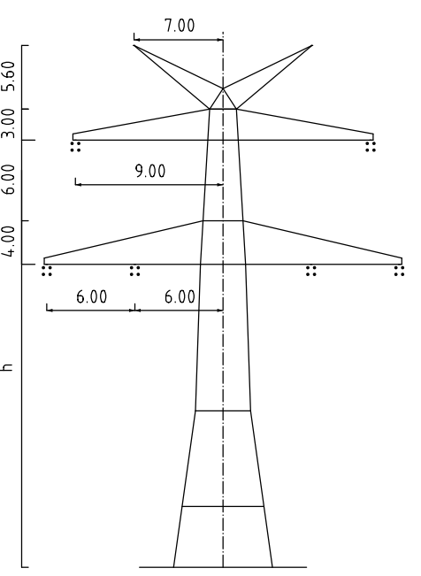
Mast Nr. 007
