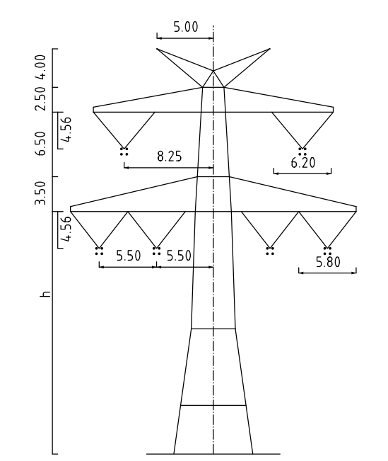
Mast Nr. 005, 006
