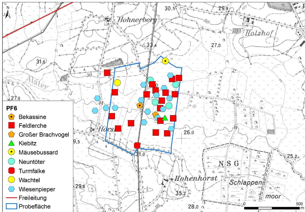
Abbildung A-12: Lage der Reviere ausgewählter Brutvogelarten, Probefläche 06 Oberalstertal.
