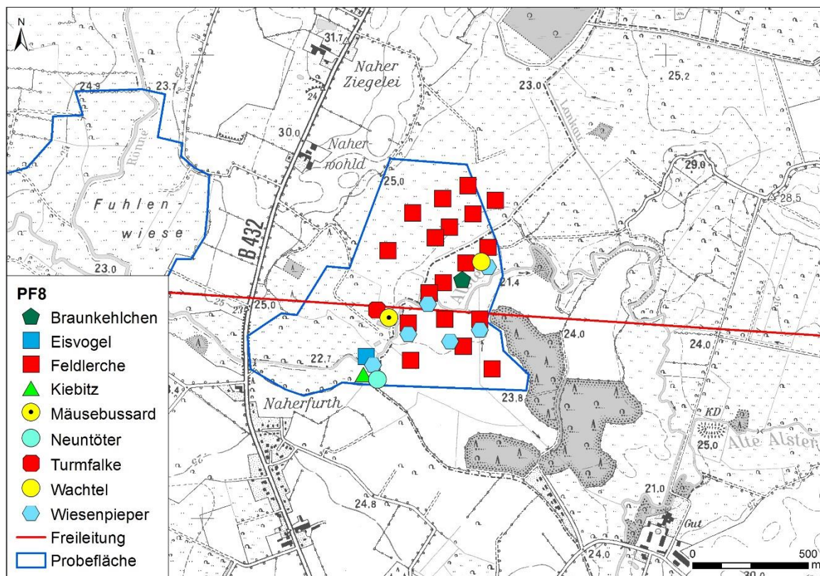
Abbildung A-14: Lage der Reviere ausgewählter Brutvogelarten, Probefläche 08 Naherfurth.
