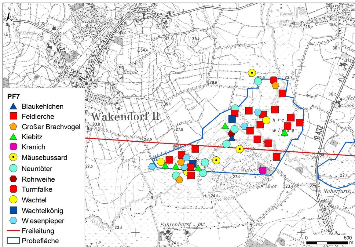
Abbildung A-13: Lage der Reviere ausgewählter Brutvogelarten, Probefläche 07 Fuhlenwiese/Wakendorfer Moor.
