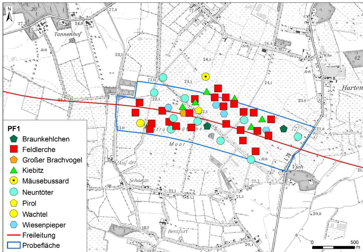
Abbildung A-7: Lage der Reviere ausgewählter Brutvogelarten, Probefläche 01 Struvenhüttener Moor.
