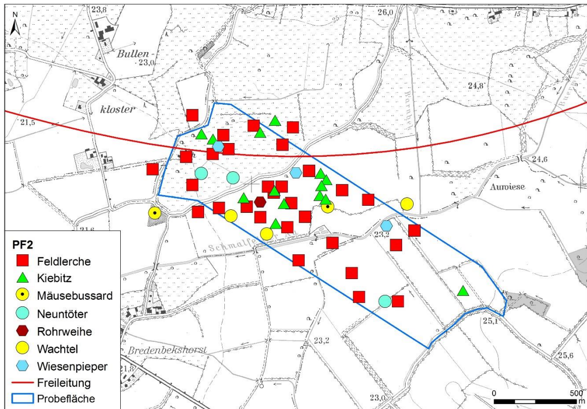
Abbildung A-8: Lage der Reviere ausgewählter Brutvogelarten, Probefläche 02 Schmalfelder Au.
