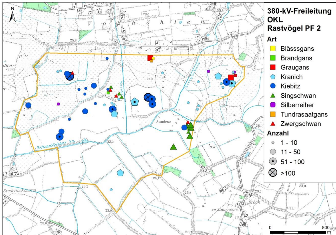
Abbildung A-2: Rastvorkommen ausgewählter Arten, Probefläche 2.
