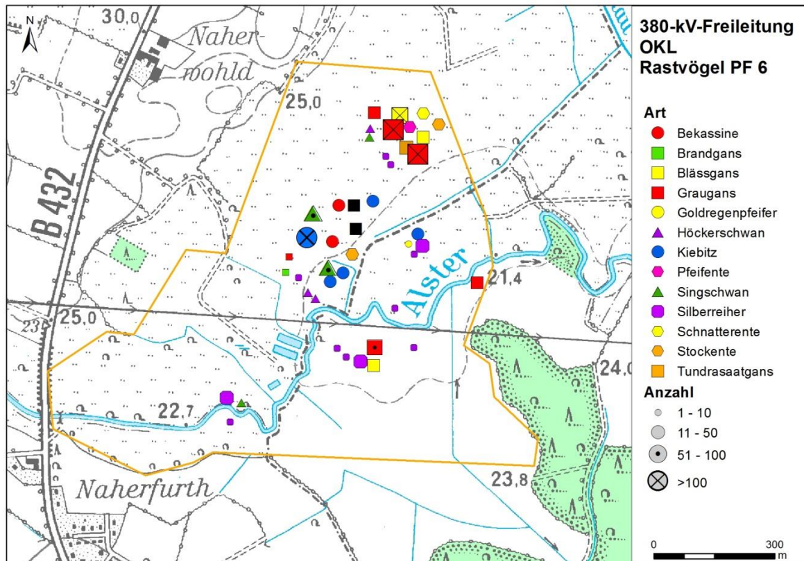
Abbildung A-6: Rastvorkommen ausgewählter Arten, Probefläche 6.
