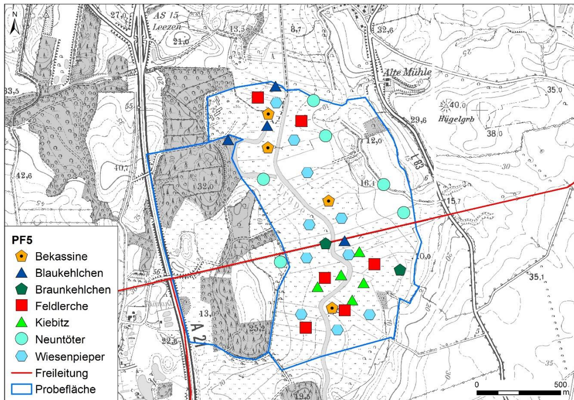
Abbildung A-11: Lage der Reviere ausgewählter Brutvogelarten, Probefläche 05 Travenbrück.
