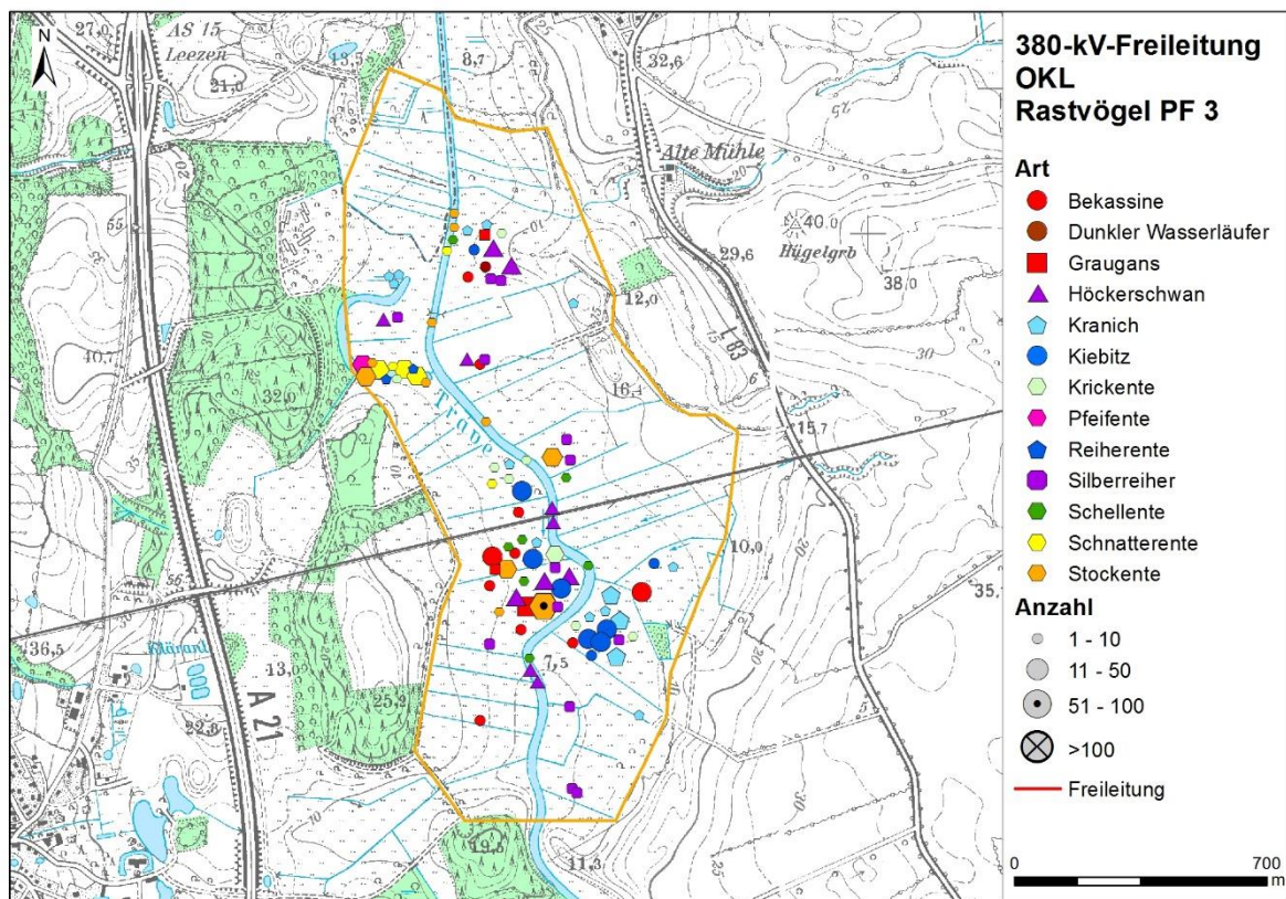
Abbildung A-3: Rastvorkommen ausgewählter Arten, Probefläche 3.
