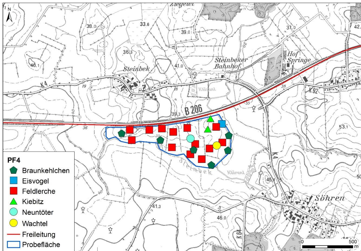
Abbildung A-10: Lage der Reviere ausgewählter Brutvogelarten, Probefläche 04 Steinbek.
