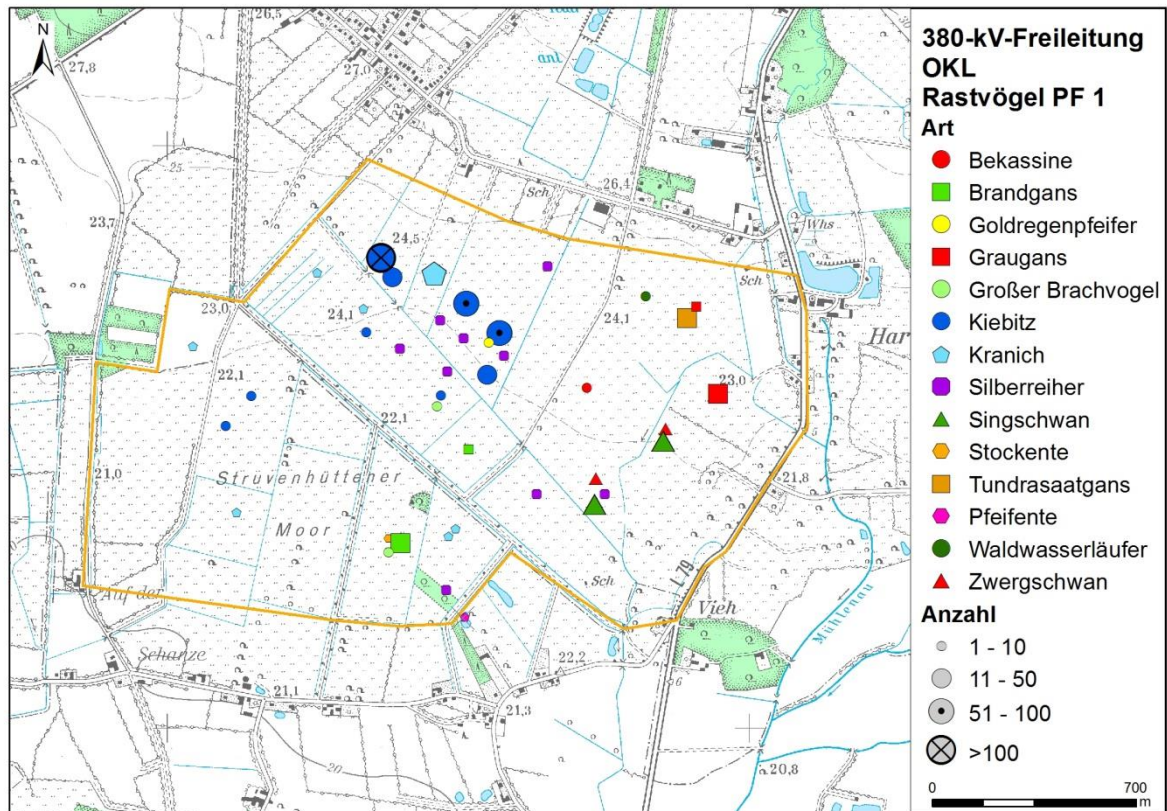
Abbildung A-1: Rastvorkommen ausgewählter Arten, Probefläche 1.
