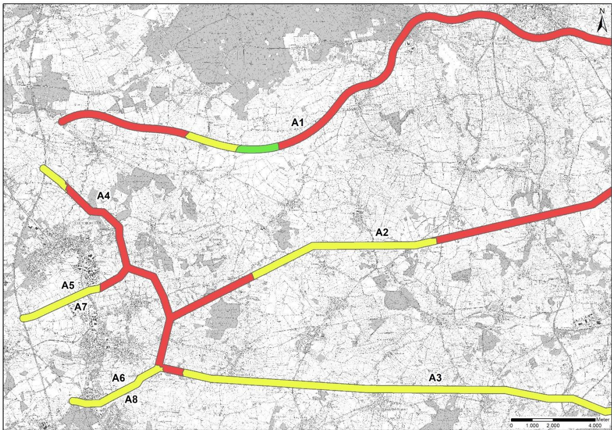
Abbildung A-15: Vorkommenswahrscheinlichkeit der Haselmaus innerhalb eines 350 m-Korridors entlang der Trassenvarianten im Westen des Betrachtungsraumes. Rot= hohe Wahrscheinlichkeit (A), gelb= mittlere Wahrscheinlichkeit (B), hellgrün= keine Habitateignung aufgrund fehlender naturräumlicher Eignung (D). Einstufungskriterien siehe Text.
