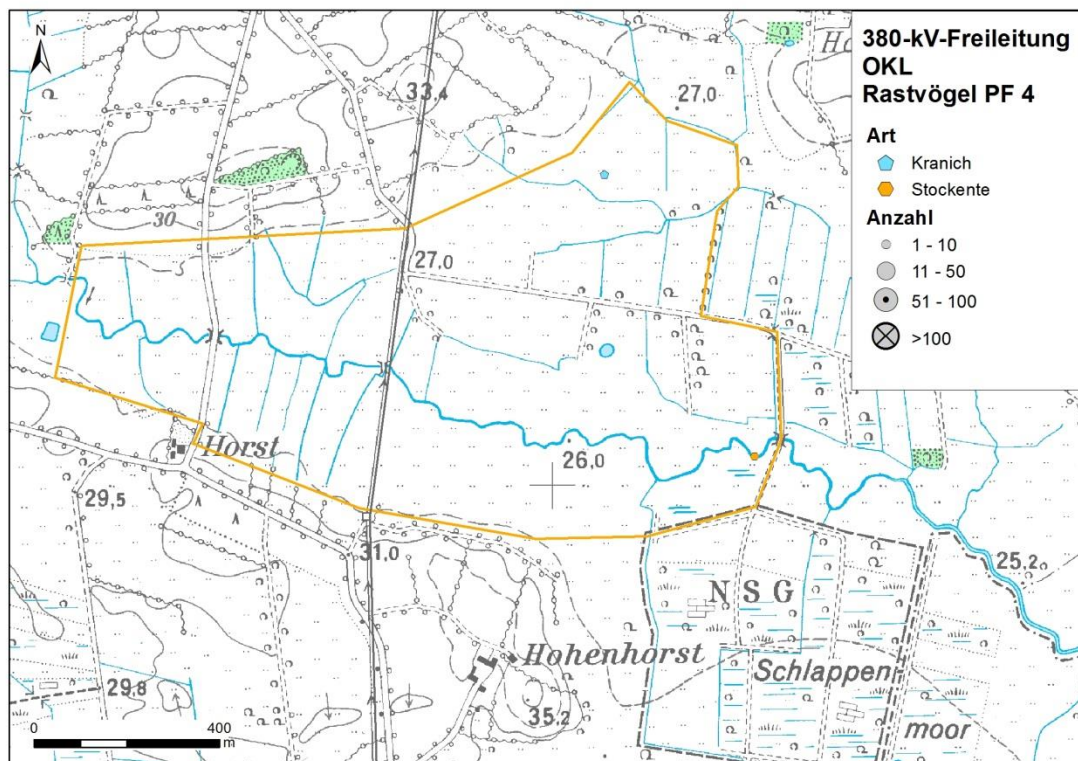
Abbildung A-4: Rastvorkommen ausgewählter Arten, Probefläche 4.
