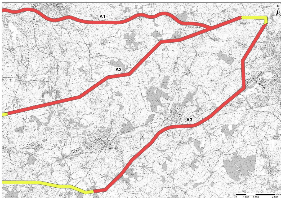
Abbildung A-16: Vorkommenswahrscheinlichkeit der Haselmaus innerhalb eines 350 m-Korridors entlang der Trassenvarianten im Osten des Betrachtungsraumes. Rot= hohe Wahrscheinlichkeit (A), gelb= mittlere Wahrscheinlichkeit (B). Einstufungskriterien siehe Text.
