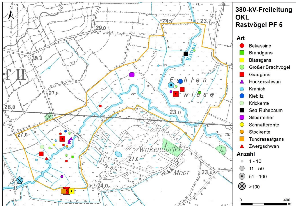
Abbildung A-5: Rastvorkommen ausgewählter Arten, Probefläche 5 (Sea Ruhebaum = Seeadler-Ruhebaum).
