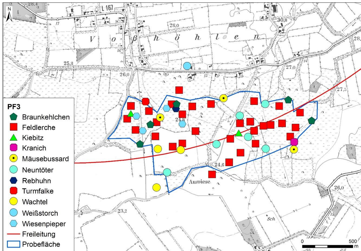
Abbildung A-9: Lage der Reviere ausgewählter Brutvogelarten, Probefläche 03 Voßhöhlen.
