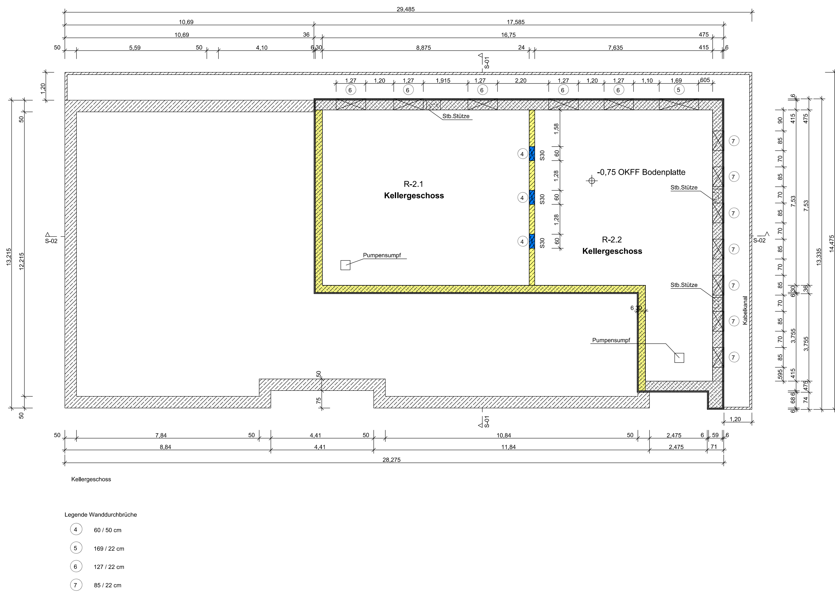
Grundriss Kellergeschoss
