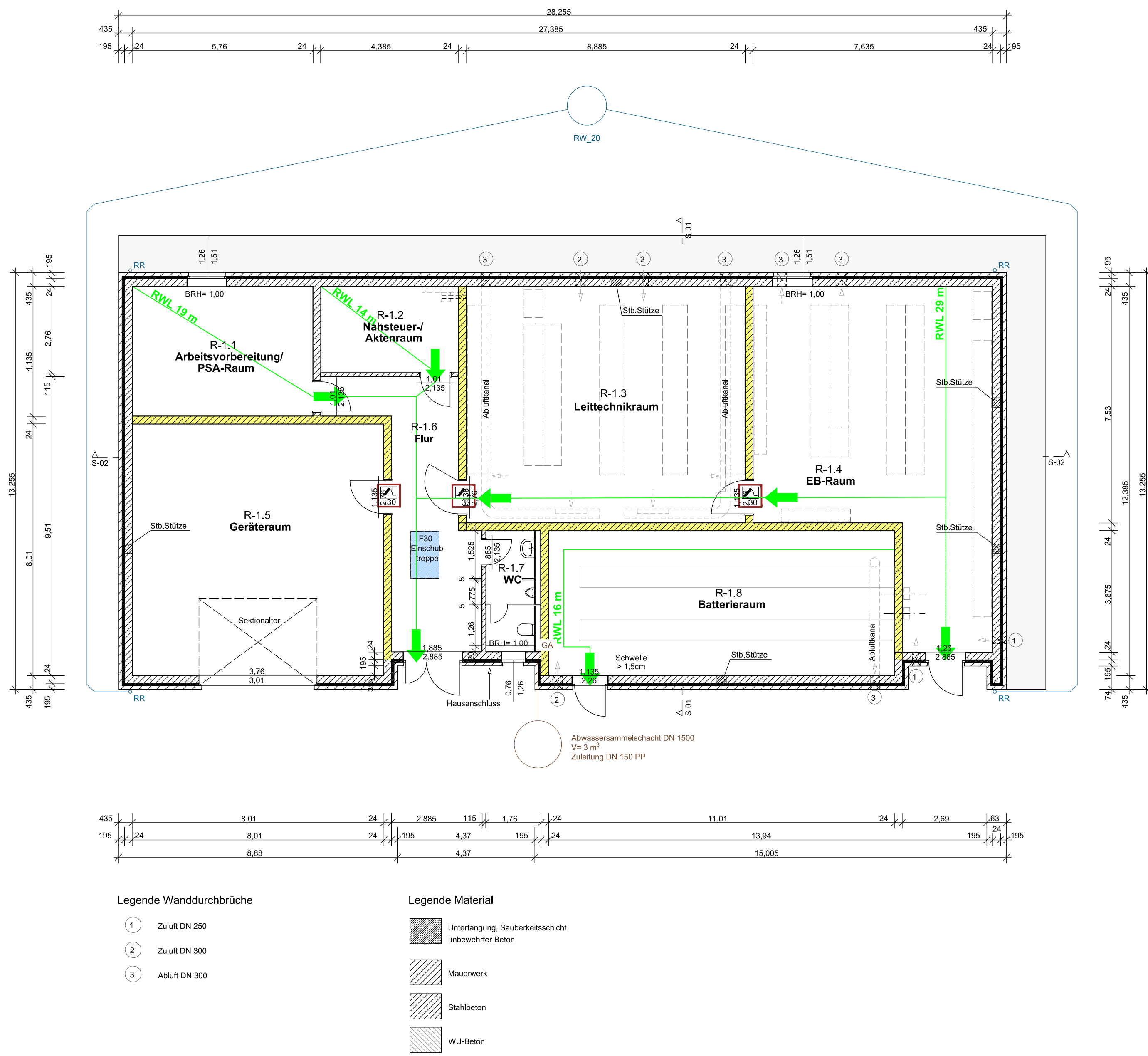
Grundriss Erdgeschoss
