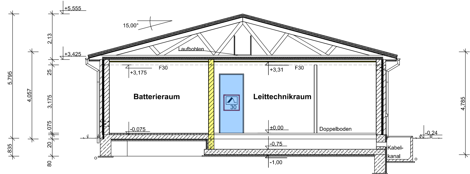
Schnitt 01-01
