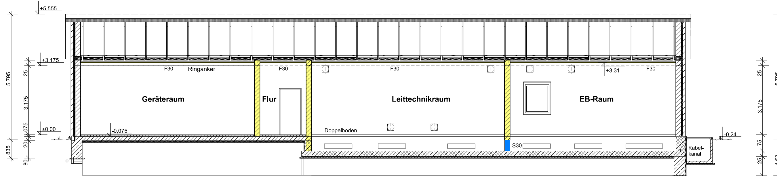
Schnitt 02-02
