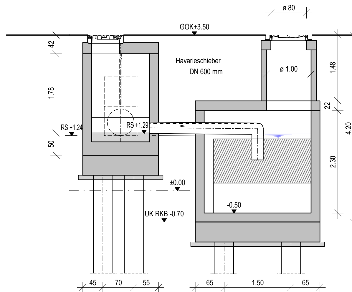
SCHNITT 3 - 3 1:50
