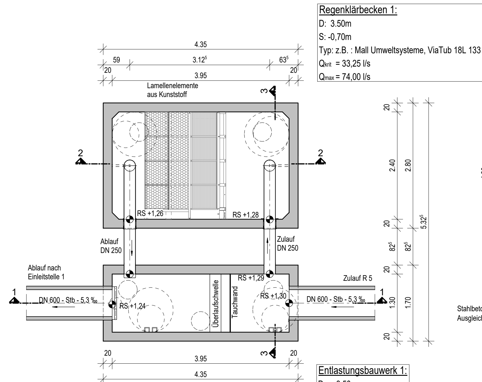
DRAUFSICHT 1:50
