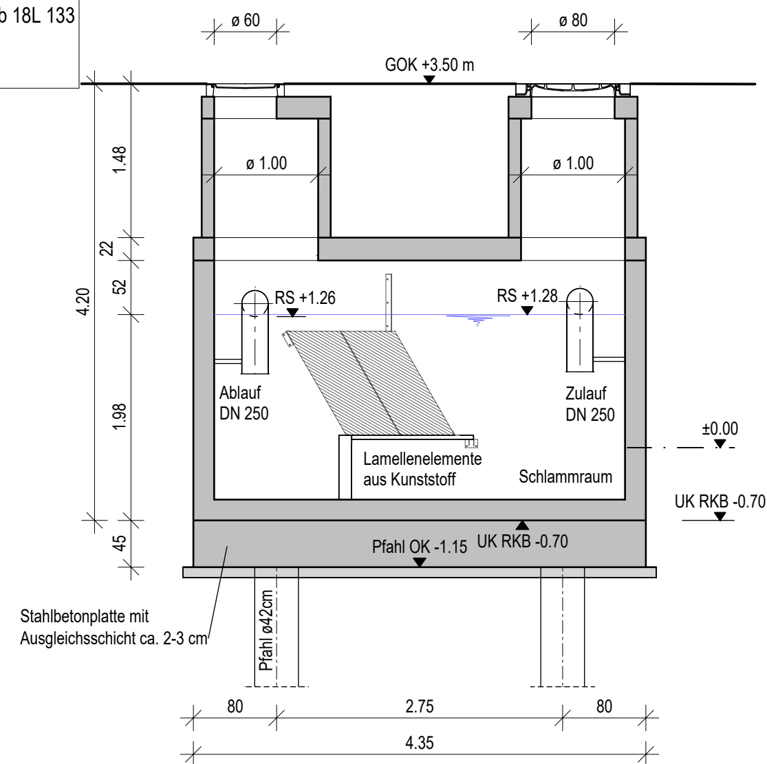
SCHNITT 2 - 2 1:50
