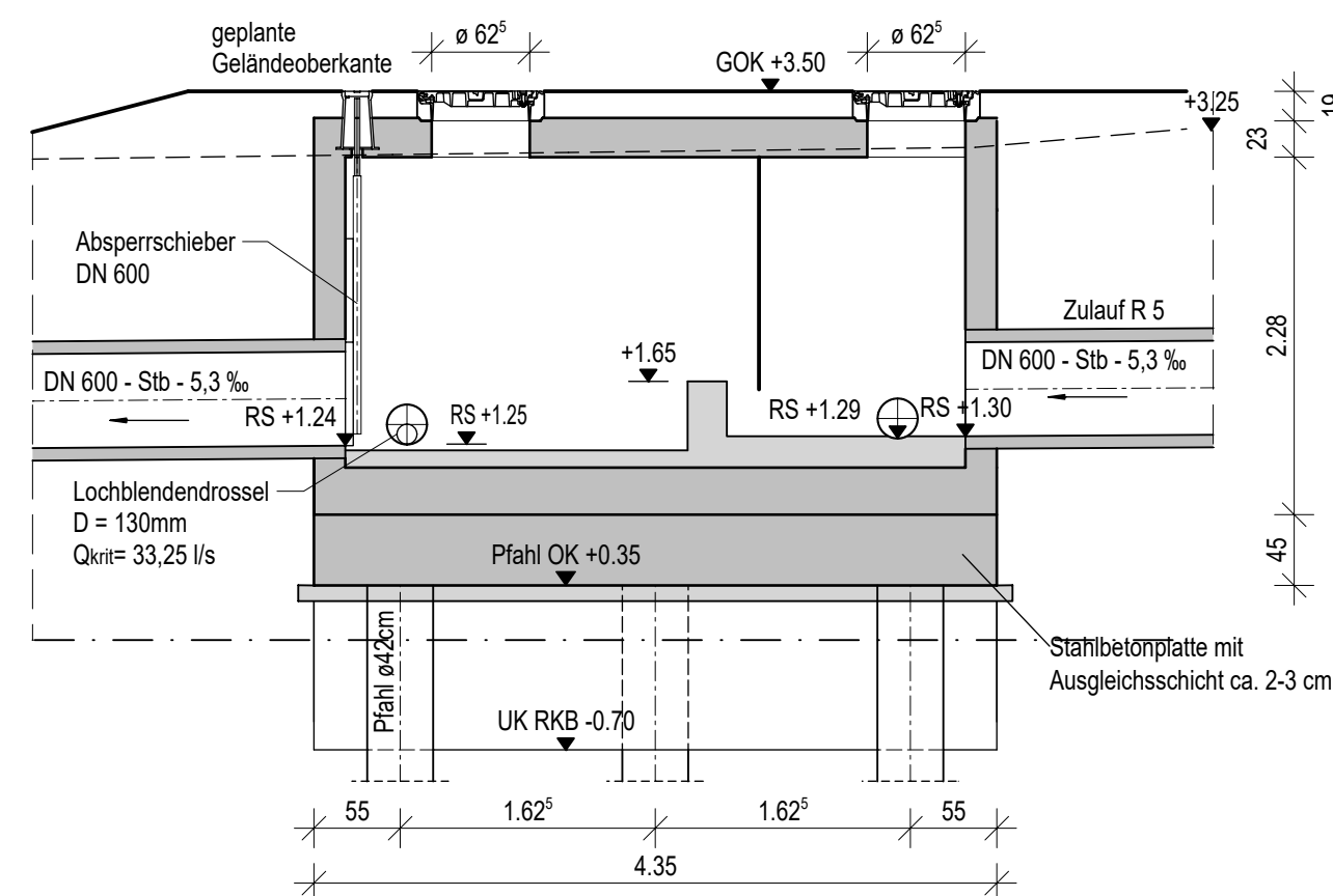
SCHNITT 1-1 1:50
