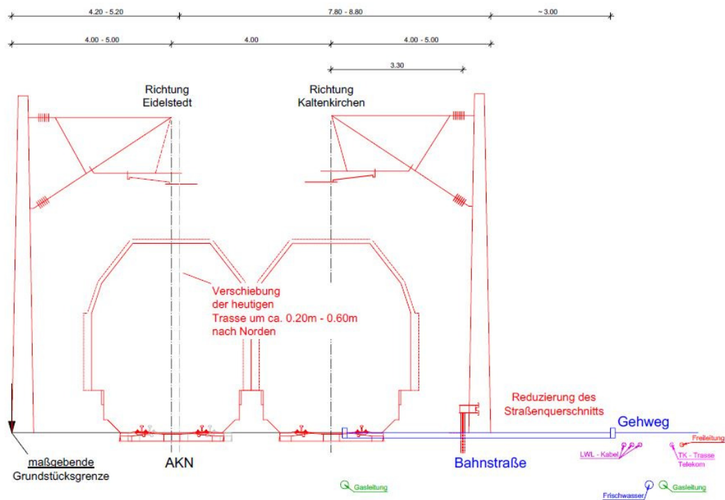
Abbildung 2: Querschnitt Variante 2
