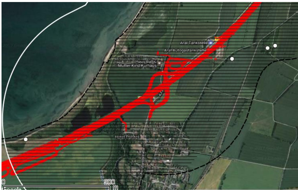
Abbildung 4-1: Neuntöttervorkommen 2016: Neuntöttervorkommen = Kreise, Untersuchungsgebiet B 207 = gestrichelte Linie, Untersuchungsraum Sundquerung = weiße Linie, und Betrachtungsraum für den Datenabgleich = schraffiert, Trasse = rot, Luftbild © 2016 Google © 2009 GeoBasis-DE/BKG
