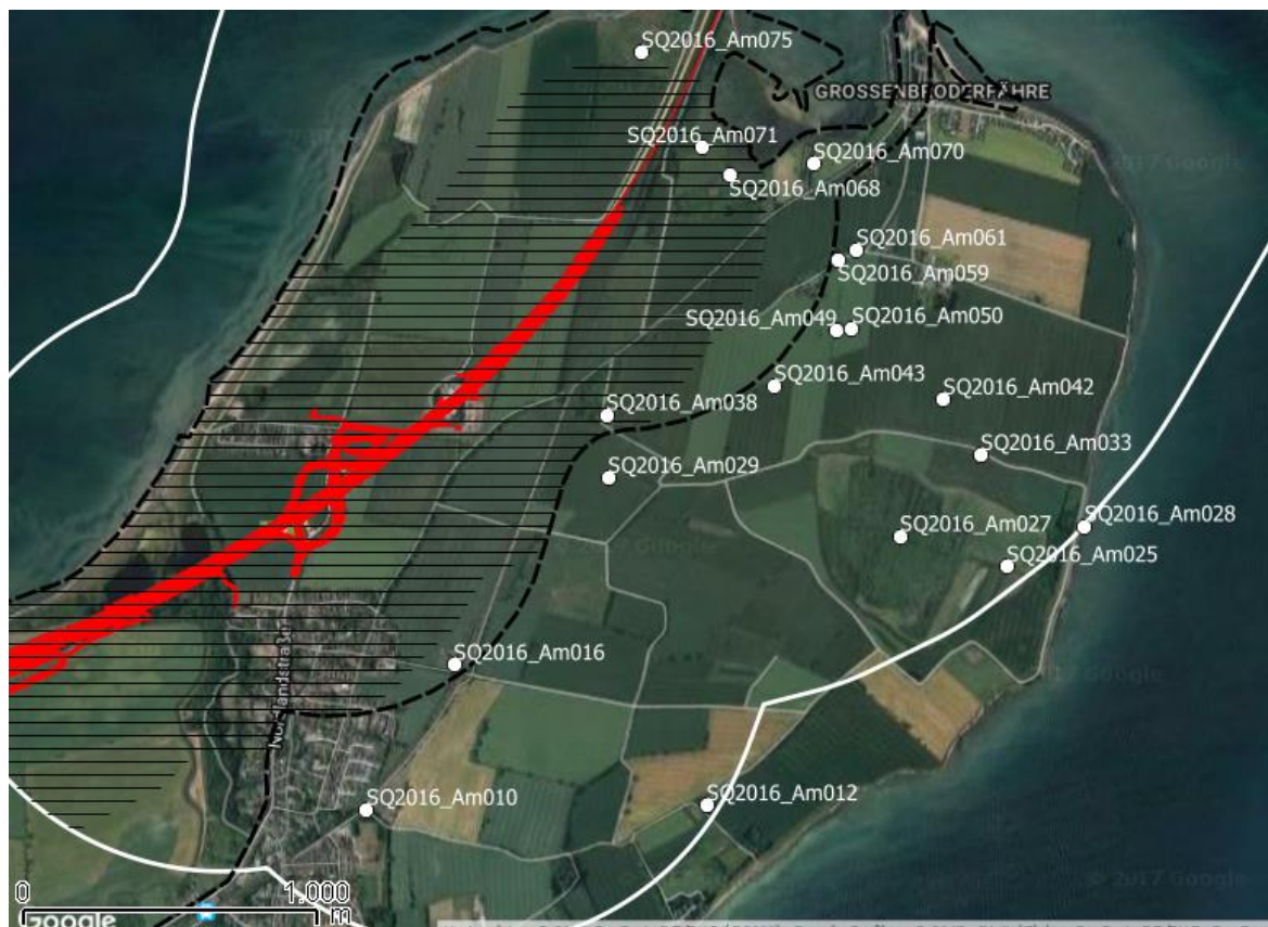
Abbildung 4-6: Kammolchvorkommen 2016 im Bereich nordöstlich Großbrode: Kammolchvorkommen ohne artenschutzrechtliche Relevanz = Kreise, Untersuchungsgebiet B 207 = gestrichelte Linie, Untersuchungsraum Sundquerung = weiße Linie, und Betrachtungsraum für den Datenabgleich = schraffiert, Trasse = rot, Luftbild © 2016 Google © 2009 GeoBasis-DE/BKG
