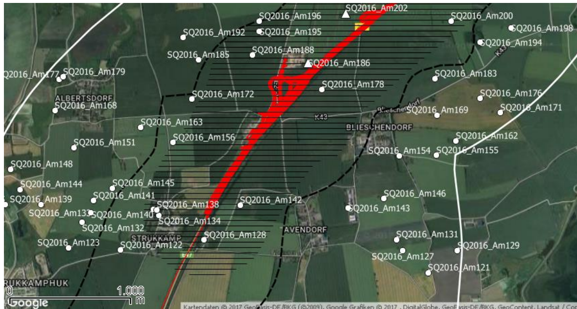
Abbildung 4-7: Kammolchvorkommen 2016 im Bereich Albertsdorf, Strukkamp, Avendorf und Blieschendorf: Kammolchvorkommen ohne artenschutzrechtliche Relevanz = Kreise, mit artenschutzrechtlicher Relevanz = Dreiecke, Untersuchungsgebiet B 207 = gestrichelte Linie, Untersuchungsraum Sundquerung = weiße Linie, und Betrachtungsraum für den Datenabgleich = schraffiert, Trasse = rot, Luftbild © 2016 Google © 2009 GeoBasis-DE/BKG
