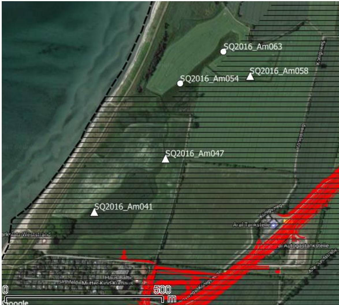
Abbildung 4-9: Kreuzkrötenvorkommen 2016: Kreuzkrötenvorkommen mit artenschutzrechtlicher Relevanz= Dreiecke, Kreuzkrötenvorkommen ohne artenschutzrechtliche Relevanz= Kreise, Untersuchungsgebiet B 207 = gestrichelte Linie und Betrachtungsraum für den Datenabgleich = schraffiert, Trasse = rot, Luftbild © 2016 Google © 2009 GeoBasis-DE/BKG
