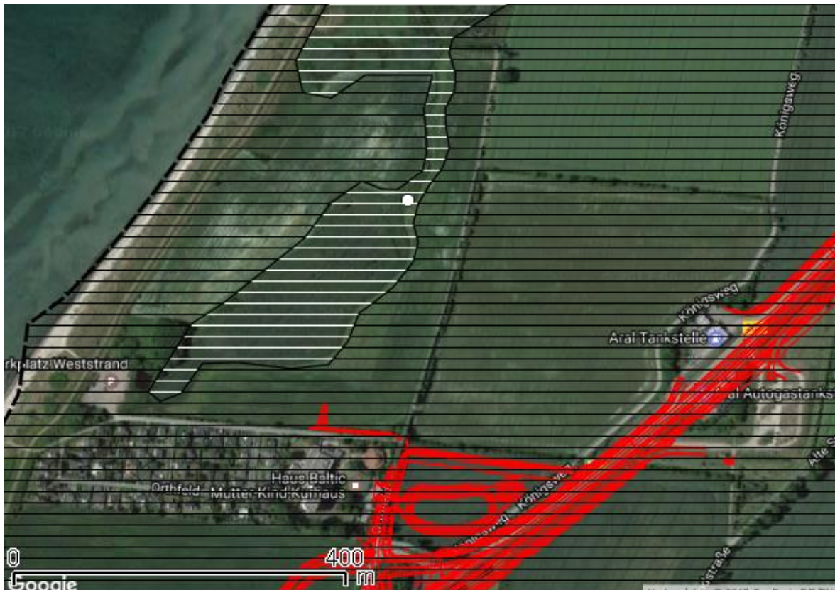
Abbildung 4-4: Rohrdommelvorkommen 2016: Fundorte = Kreise, Niederungsbe- reich = weiß schraffiert, Untersuchungsgebiet B 207 = gestrichelte Linie und Be- trachtungsraum für den Datenabgleich = schwarz schraffiert, Trasse = rot, Luftbild © 2016 Google © 2009 GeoBasis-DE/BKG
