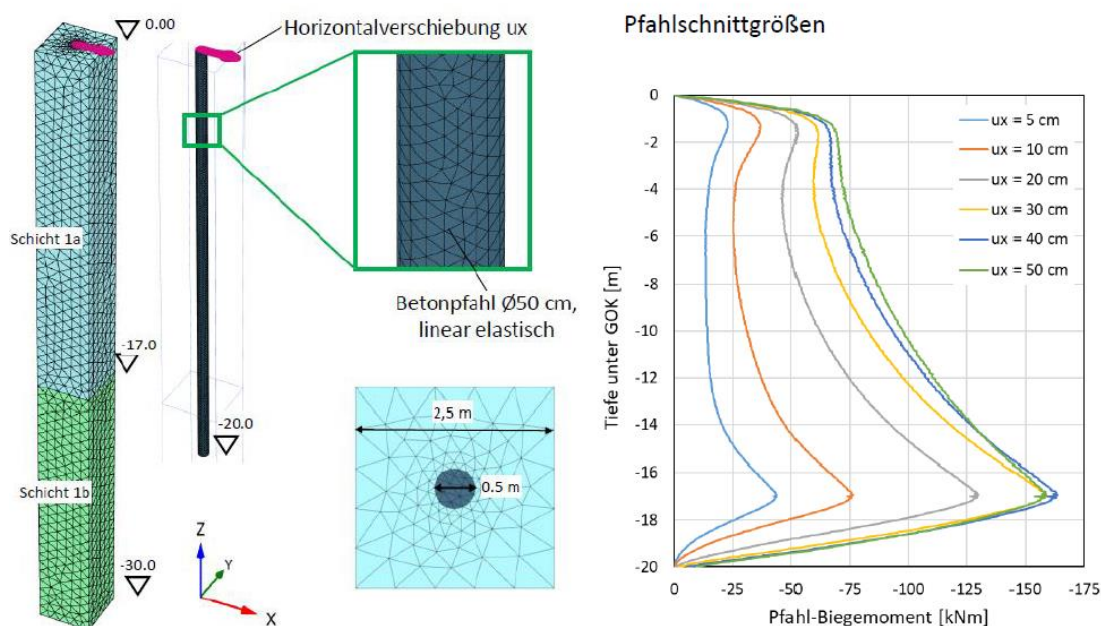
Bild 2-2 Ergebnis FEM-Berechnung: Biegemomente in einem Beton-Rammpfahl mit Durchmesser 50 cm. Links: System und Abmessungen. Rechts: Verlauf der Pfahlbiegemomente bei eingeprägten Pfahlkopfverschiebungen zwischen 5 cm und 50 cm
