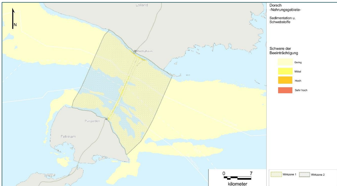
Abbildung 8-160 Darstellung der Schwere der Beeinträchtigung verursacht durch den Wirkfaktor Sedimentation und Schwebstoffe für den Absenktunnel
