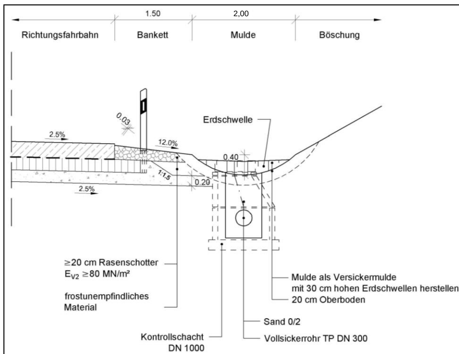
Bild 2: Entwässerungsdetail – modifiziertes Mulden-Rigolen-System
