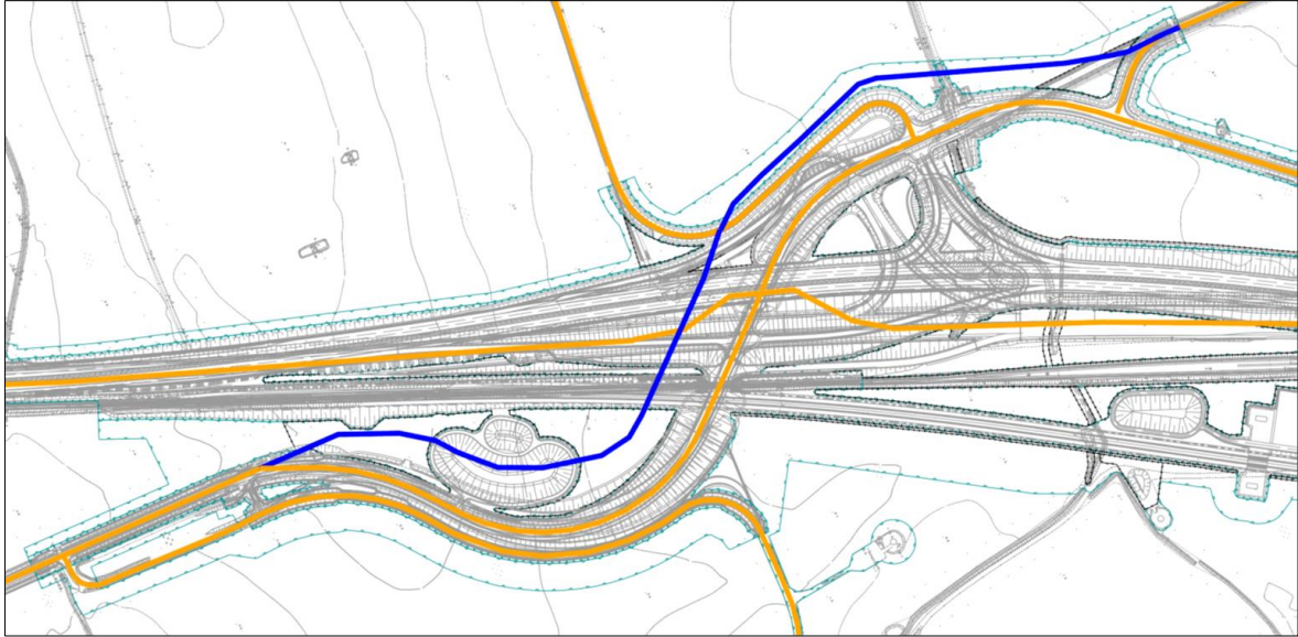
Abb. 4.18: Rückbau temporäre Umleitung K49
