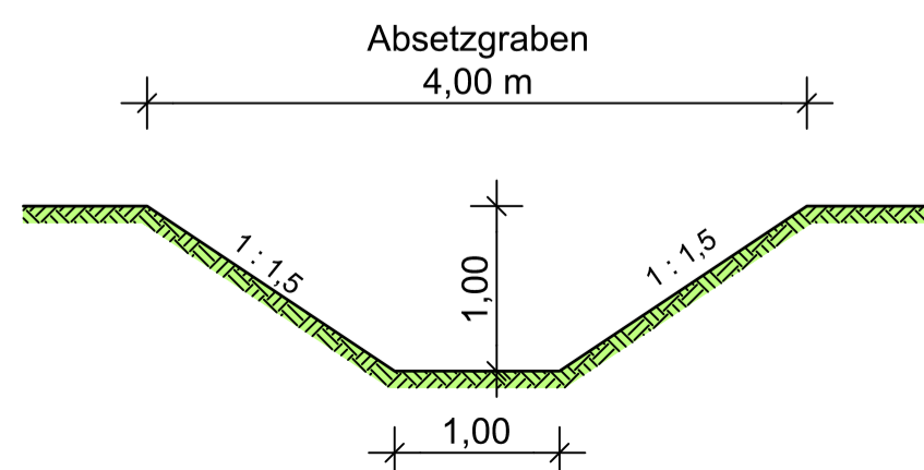
SCHNITT A-A 1:50
