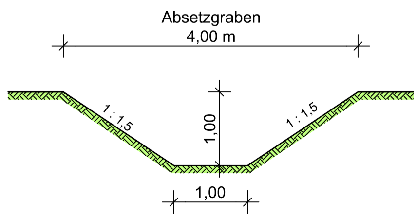
SCHNITT A-A 1:50
