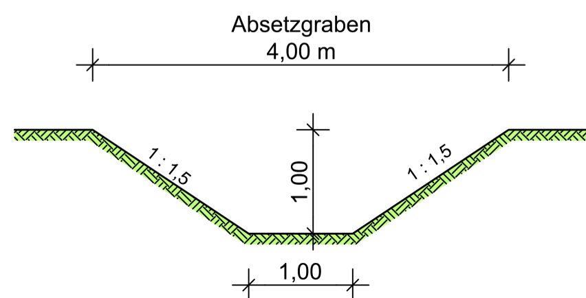
SCHNITT A-A 1:50
