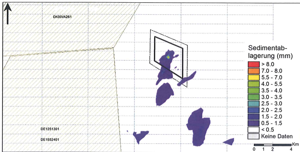
Abbildung 3-2: Modellerte maximale, vorübergehende Sedimentablagerung der Korngröße < 63 µm für ein ganzes Modelljahr (in mm, Referenzjahr 2005).
