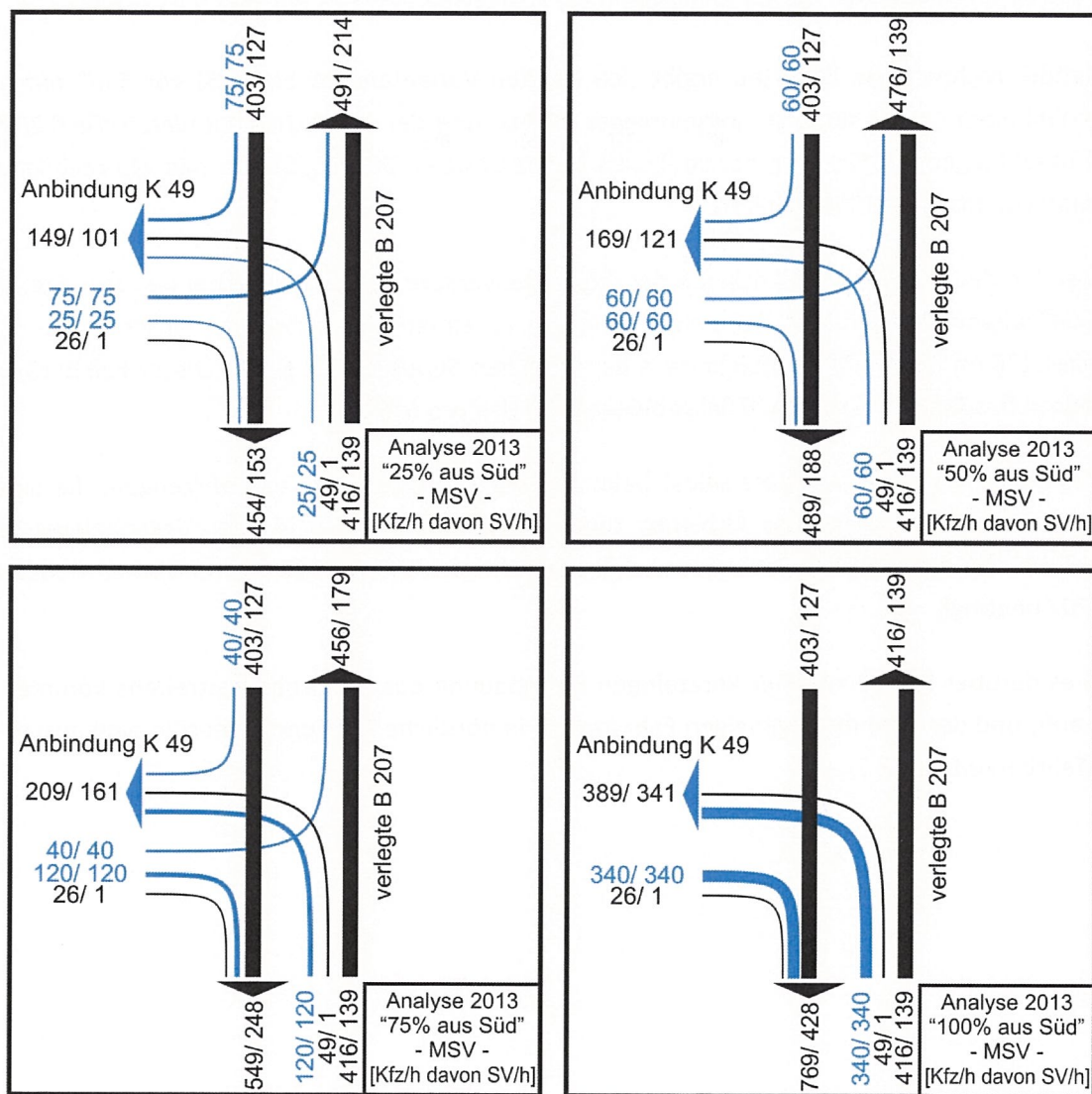
Bild 5.2: verträgliche Verkehrsverteilung (MSV)
