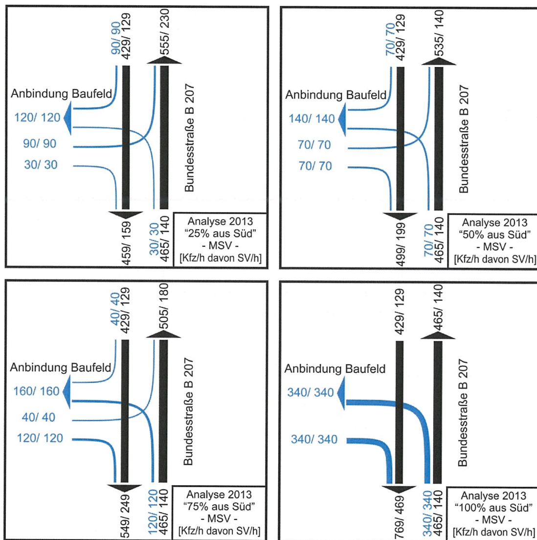
Bild 4.2: verträgliche Verkehrsverteilung (MSV)
