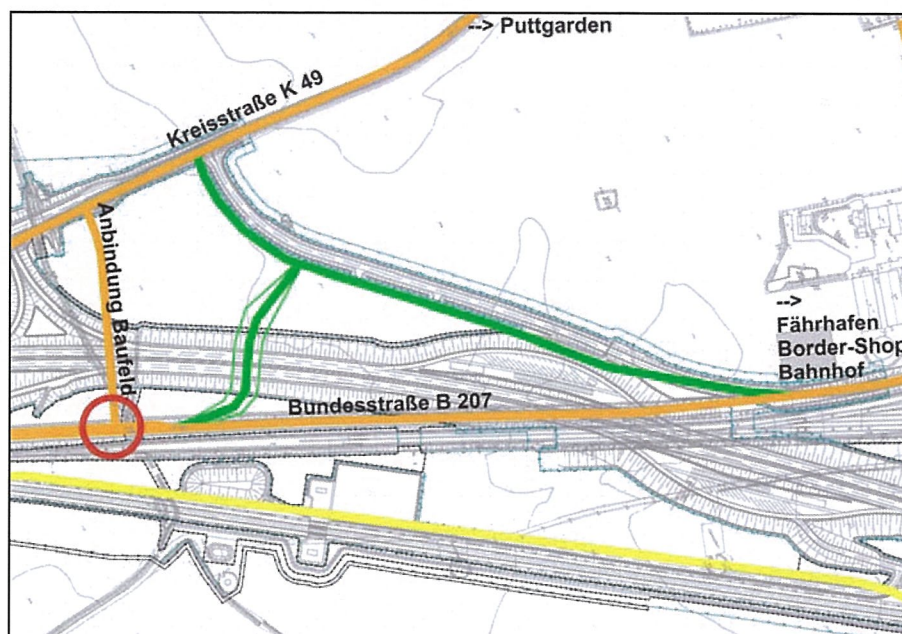
Bild 4.1: Bau Umleitung B 207 – Anschluss an Hafen
